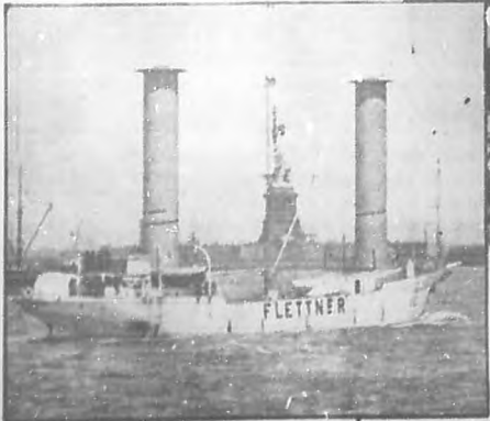
Momento que pasa ante la estatua de la Libertad, de New York, el buque-rotor "Baden-Baden", el cual está movido por un nuevo sistema de locomoción, inventado por Anton Flettner.
