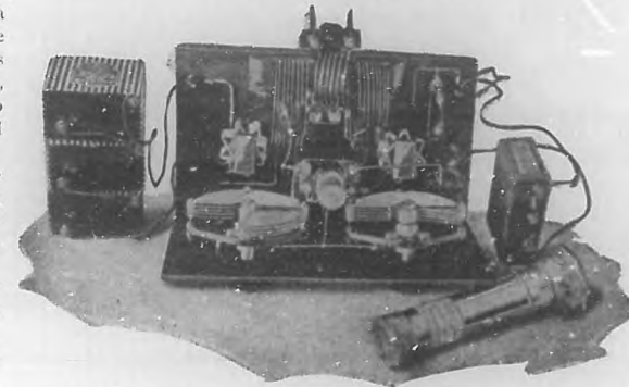
He aquí la vista completa del transmisor Miniatura, incluso su provisión de fuerza. Compárese su tamaño con la lámpara de bolsillo que se puede ver al lado de dicho aparato.
